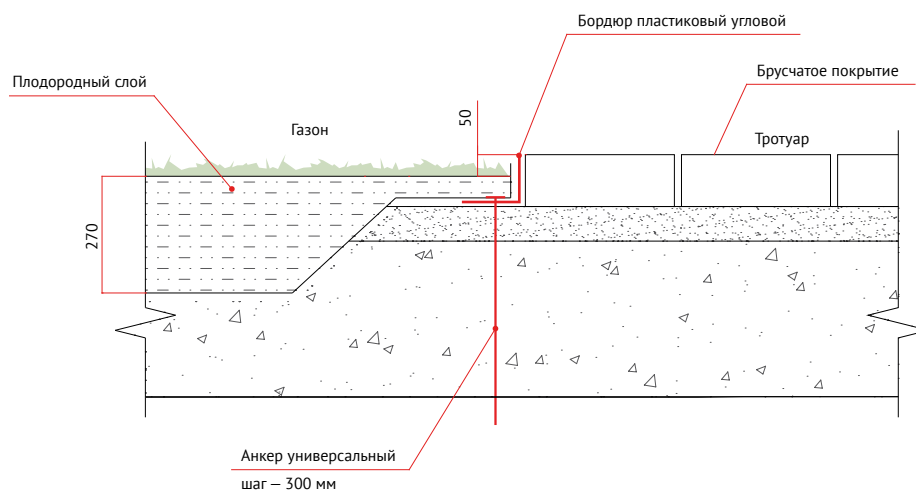
Узел 8. Сопряжение с использованием пластикового борта
